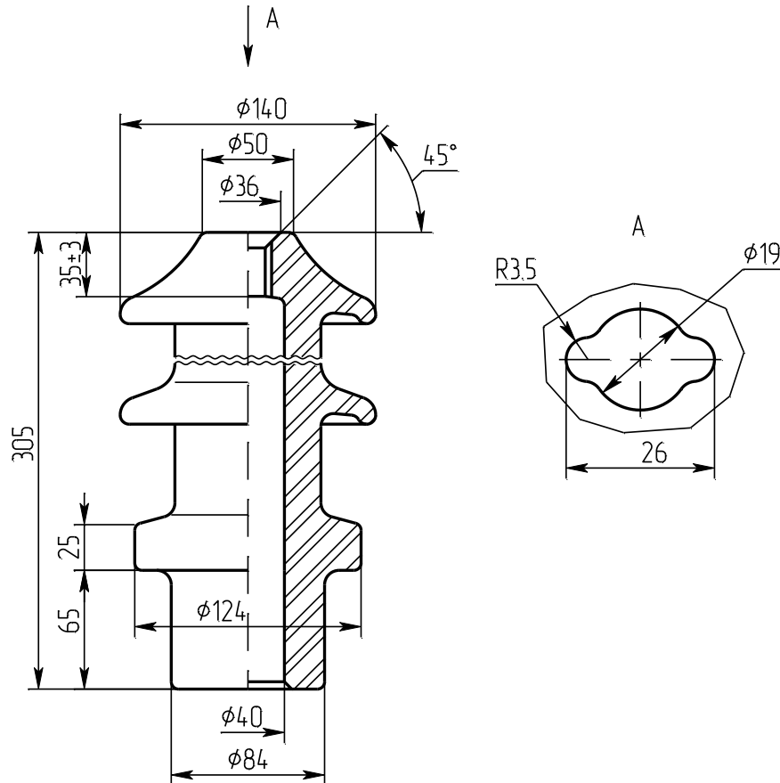
ИПТ-10/400 Б 01 чертеж ИВЕЮ.757524.048 креслення
